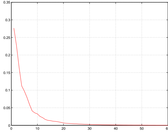
Figure 4.2: Top 60 Eigenvalues in Y -space
